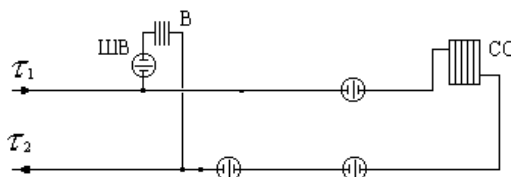
Рисунок 5. Схема «Потребитель с непосредственным присоединением СО»
