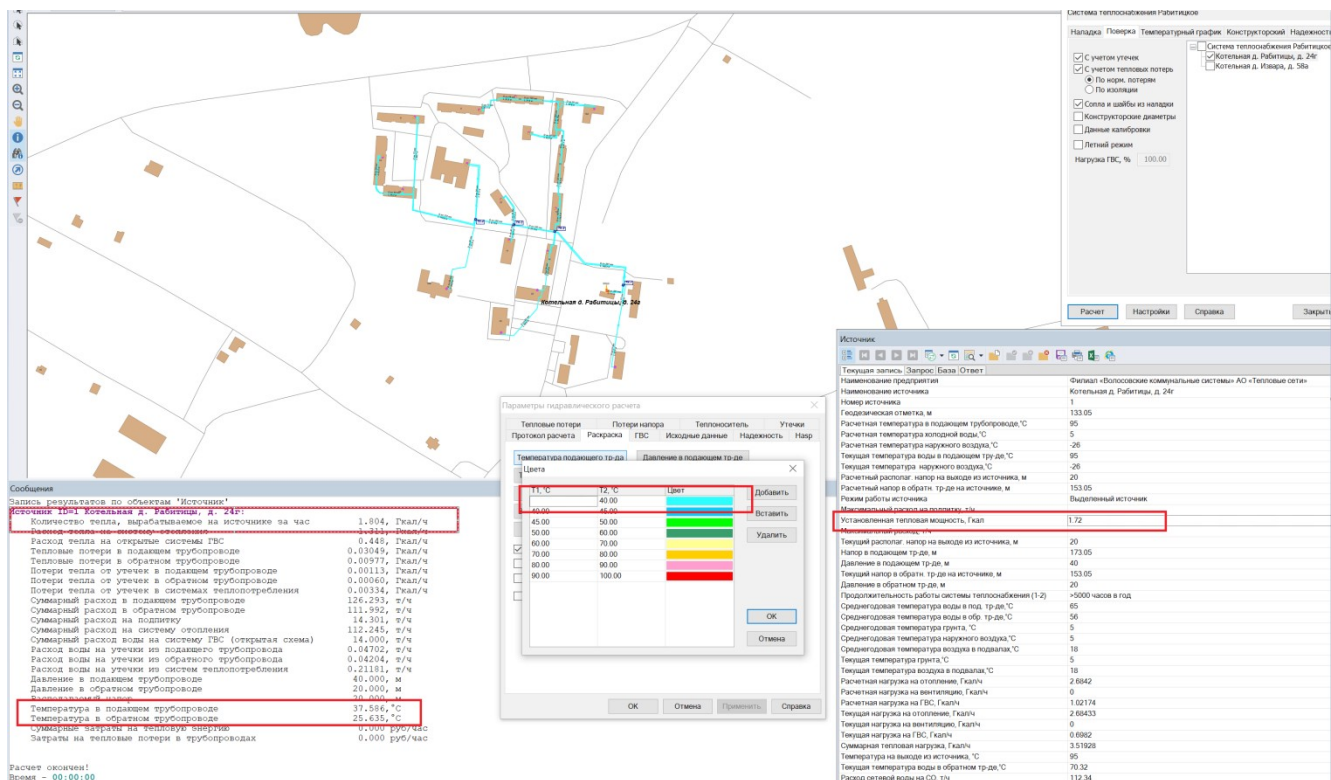
Рисунок 12. Результаты аварийного моделирования, связанного с отключением установленных котлов
